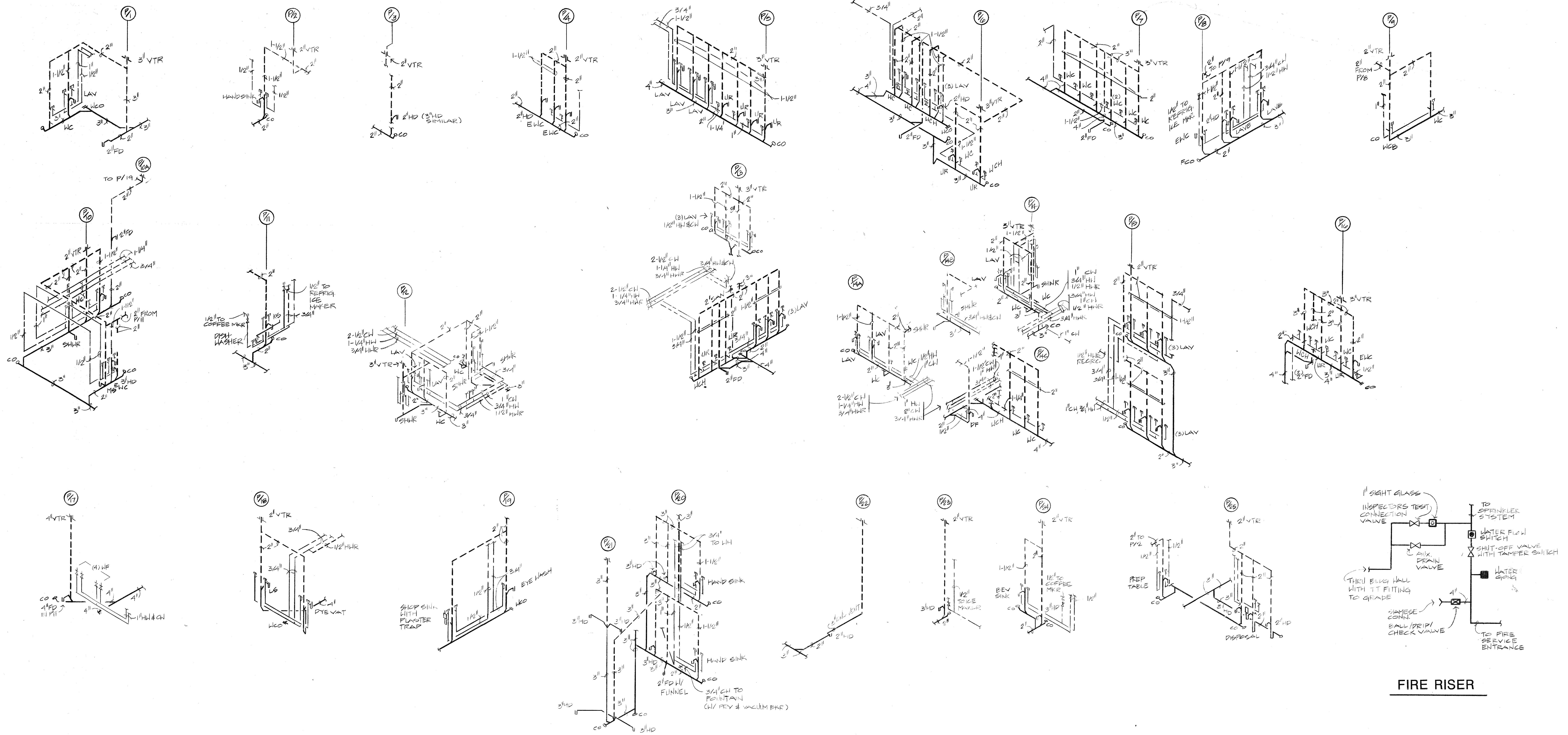
PLUMBING RISERS
