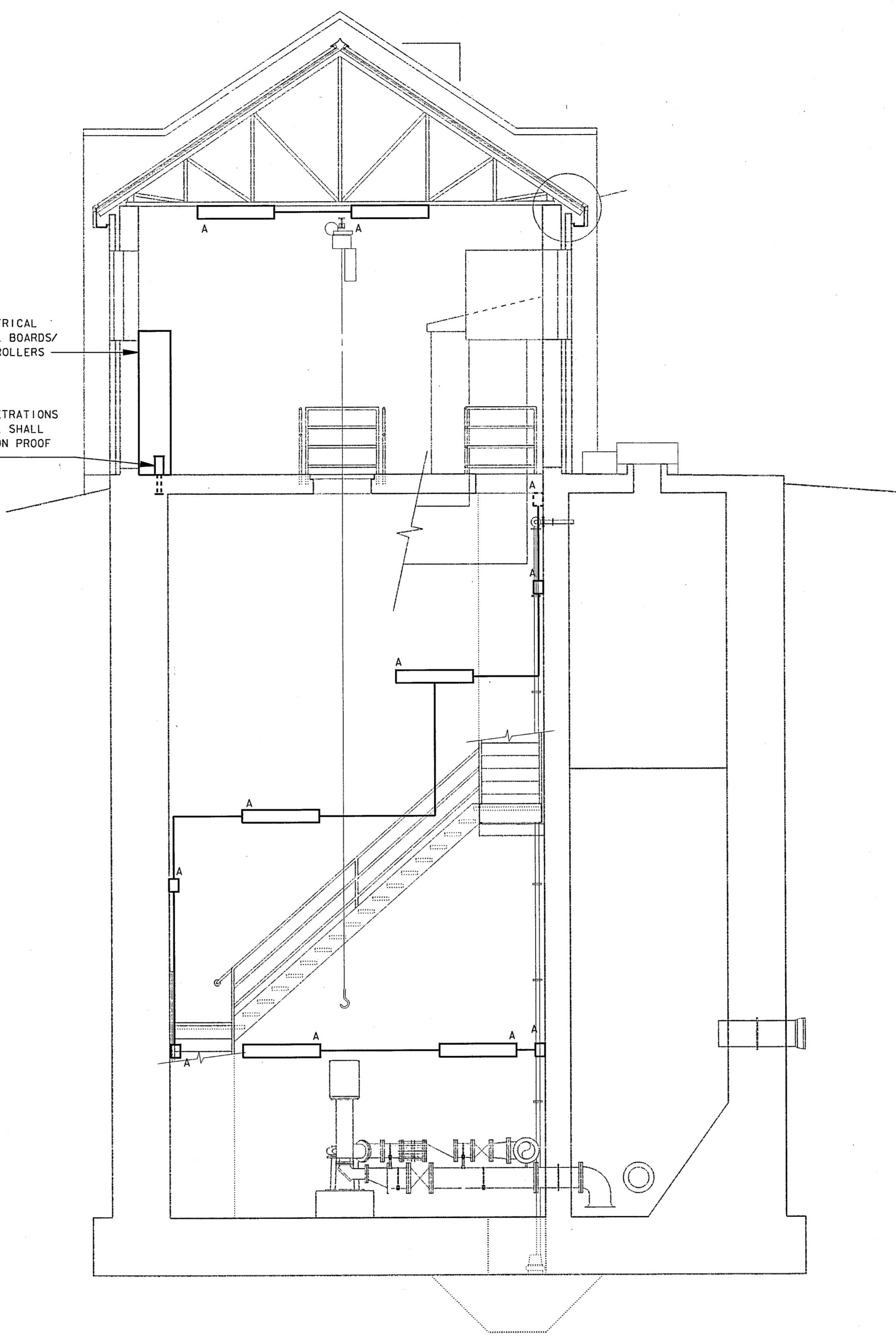
B SECTION SCALE: 1/4" = 1'-0"
