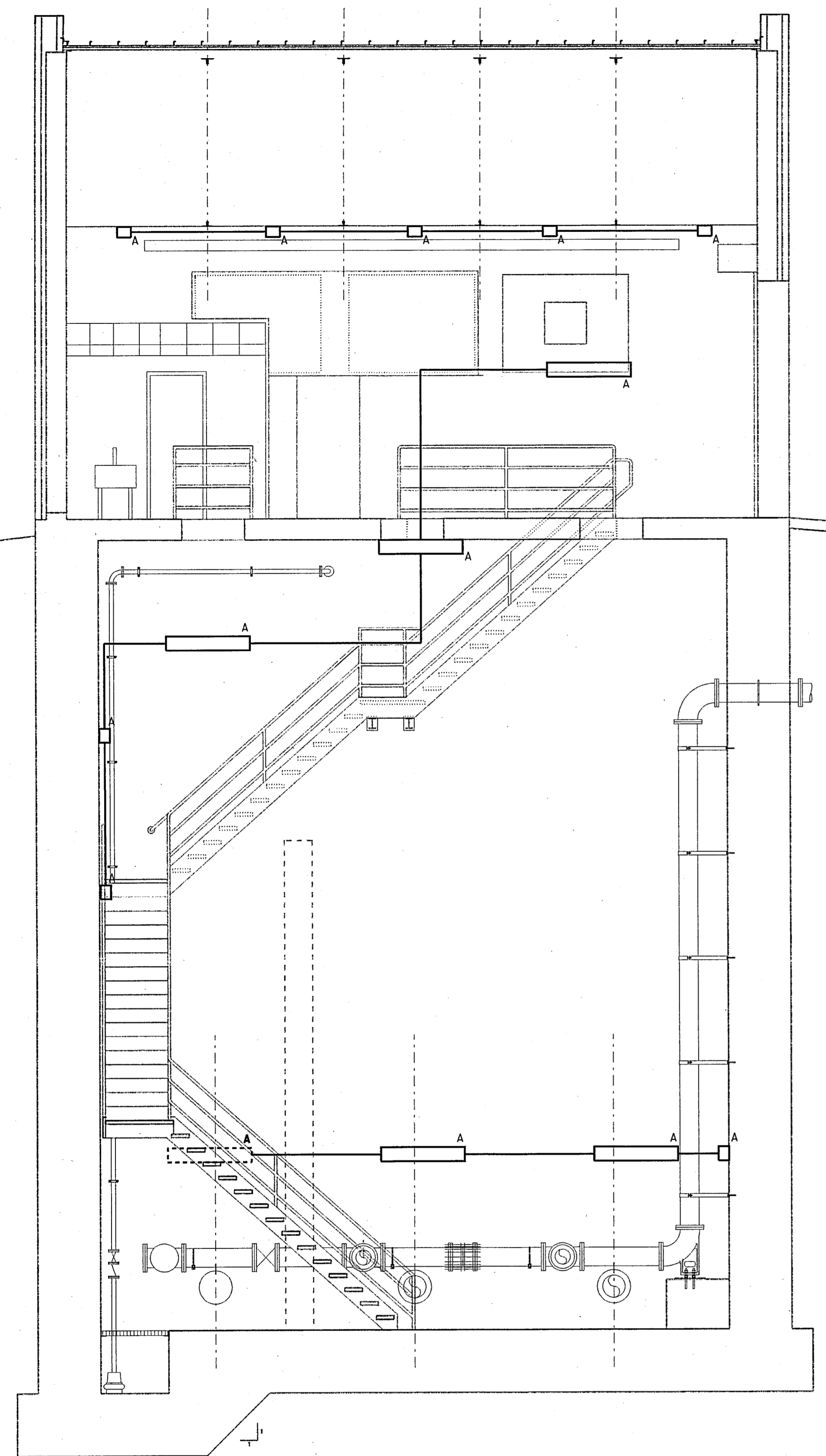
A SECTION SCALE: 1/4" = 1'-0"
