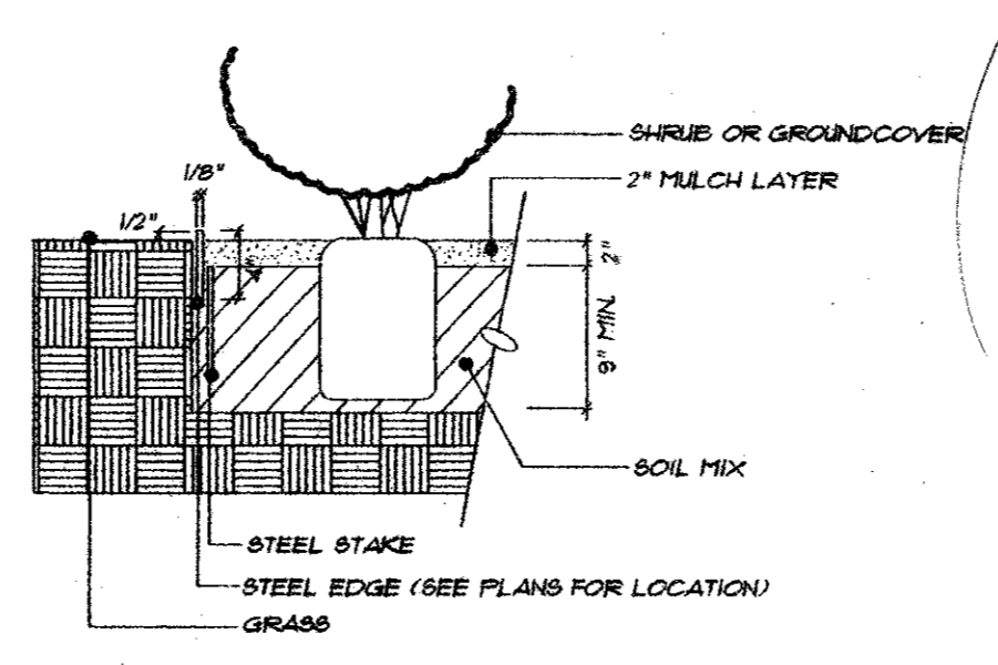
BED-PREP W/ STEEL EDGE N.T.S.
