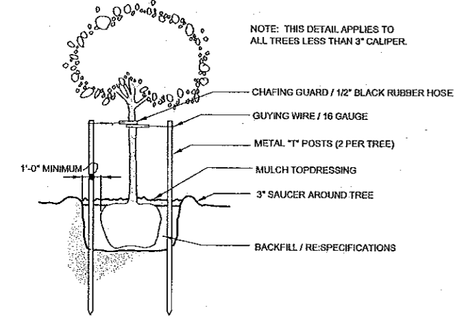
B TREE STAKING DETAIL SCALE: N.T.S.
