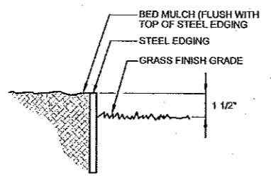
C STEEL EDGING SCALE: N.T.S.
