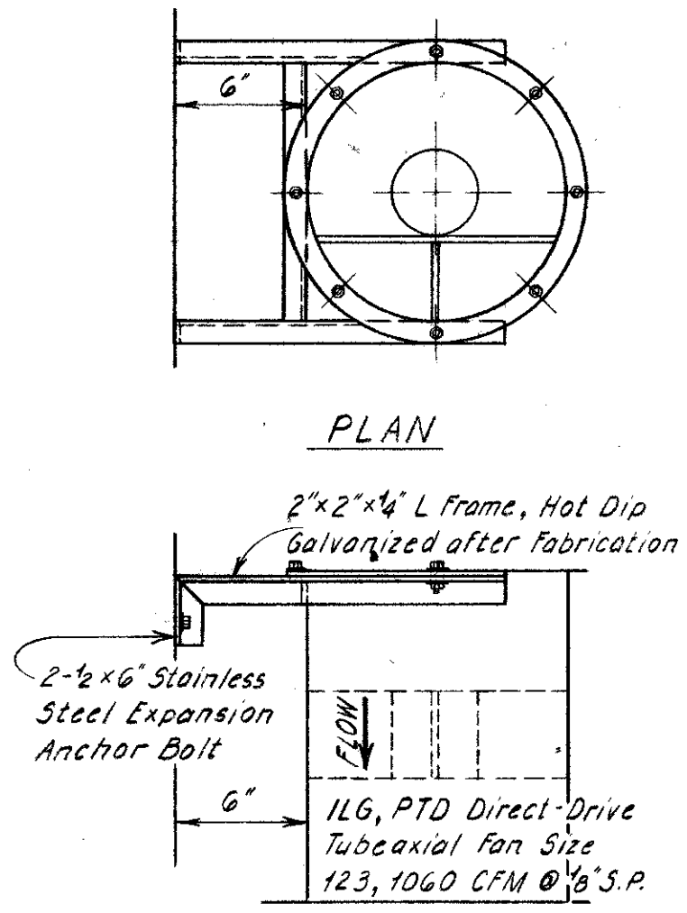
FAN INSTALLATION 1/2"=1'-0"
