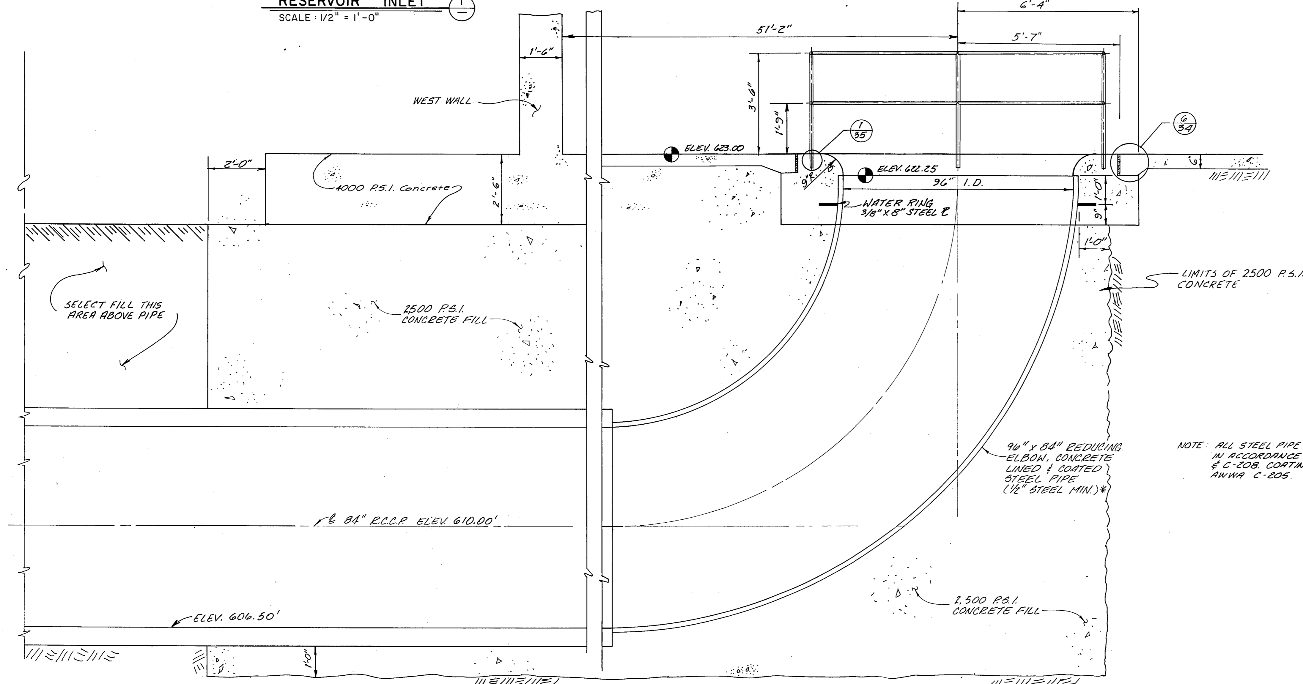
SECTION SCALE: 1/2" = 1'-0"
