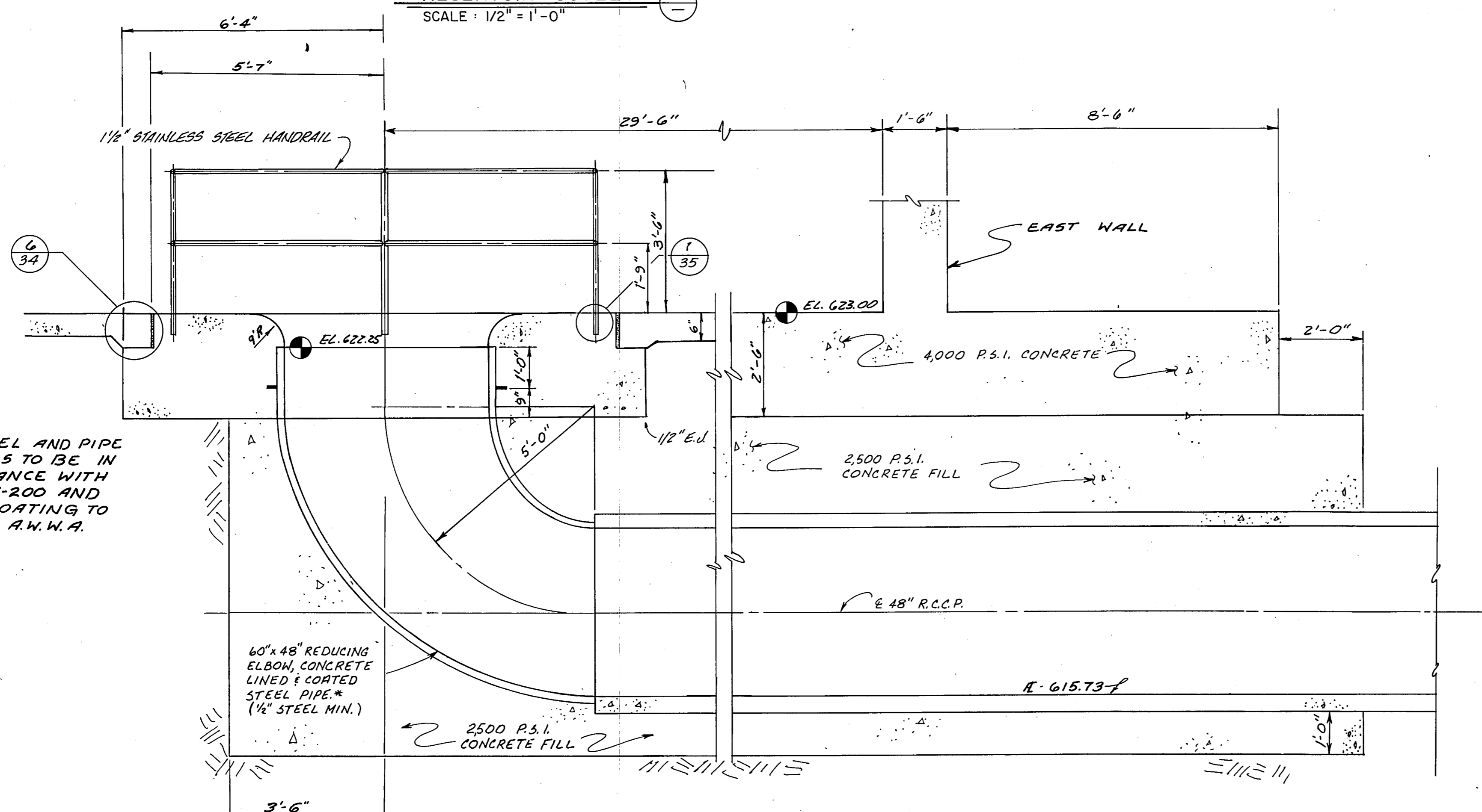
SECTION SCALE: 1/2" = 1'-0"
