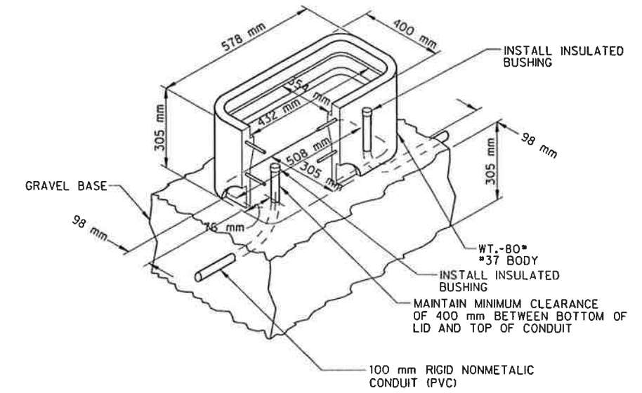
PULL BOX DETAIL N.T.S.
