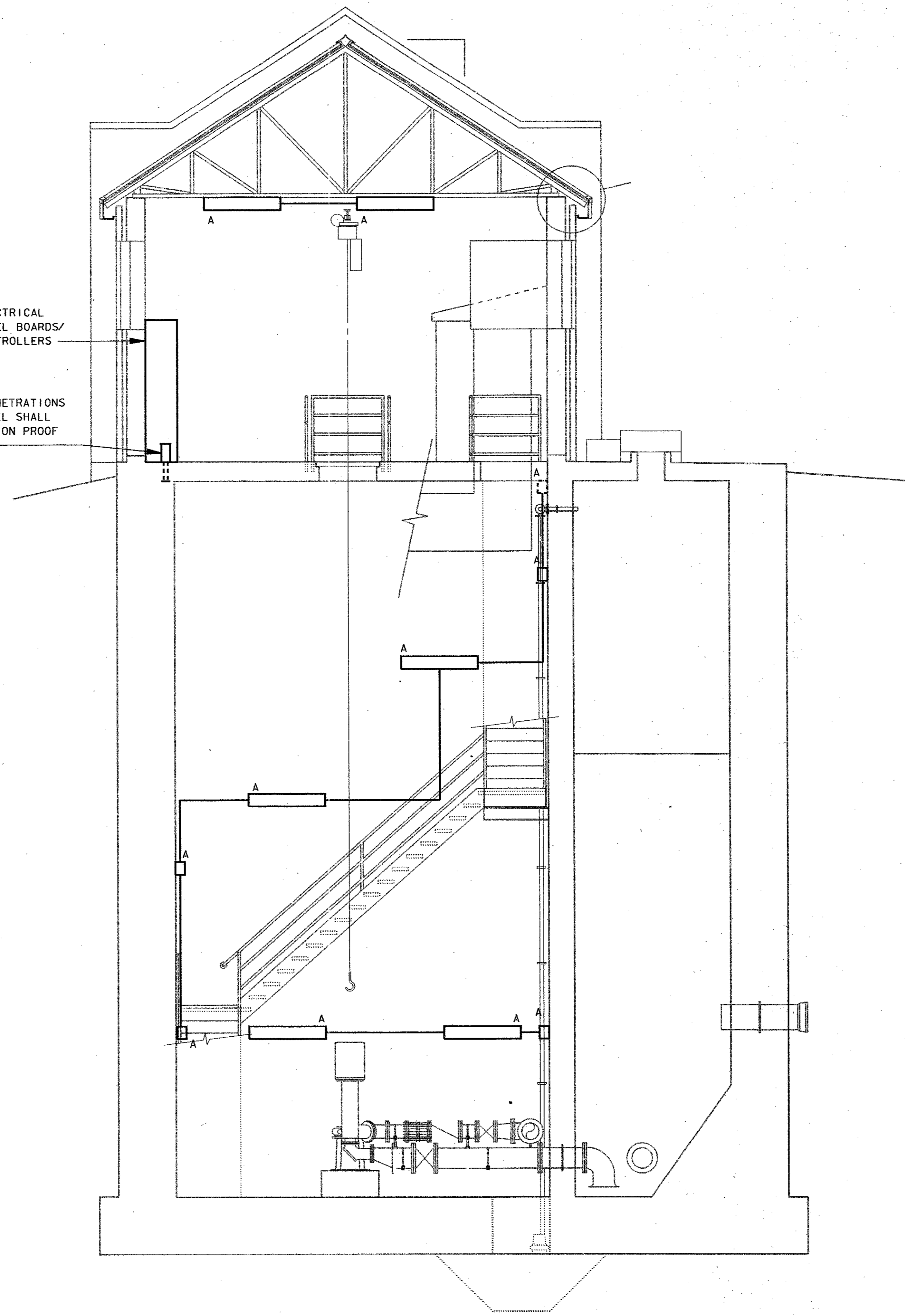
B SECTION SCALE: 1/4" = 1'-0"
