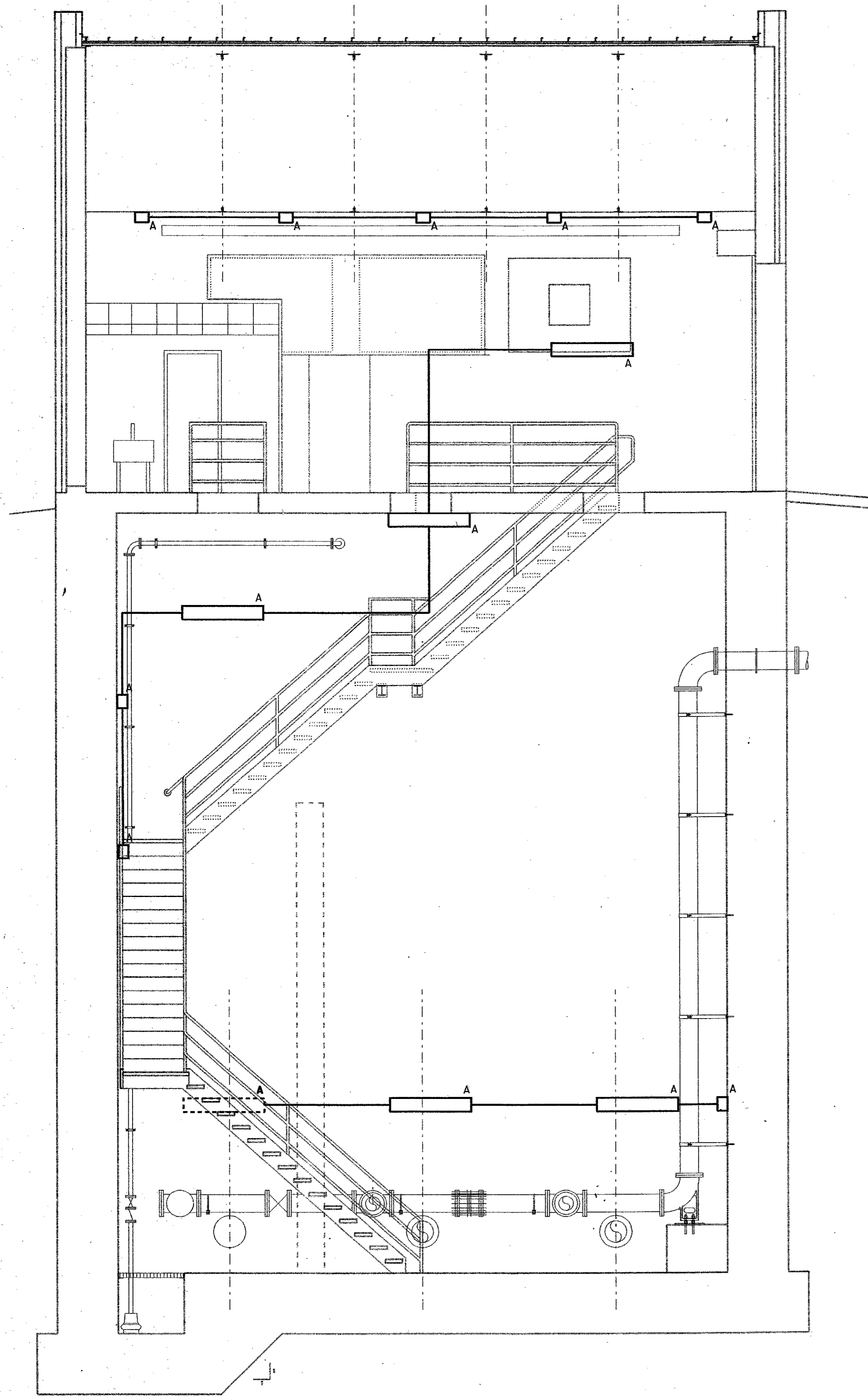
A SECTION SCALE: 1/4" = 1'-0"
