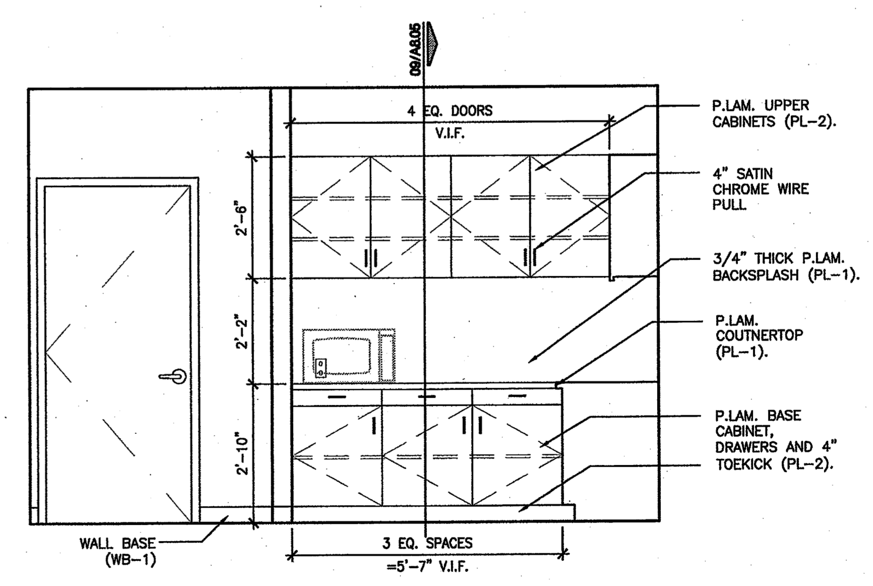
08 RECEPTION ELEV. SCALE: 1/4" = 1'-0"
