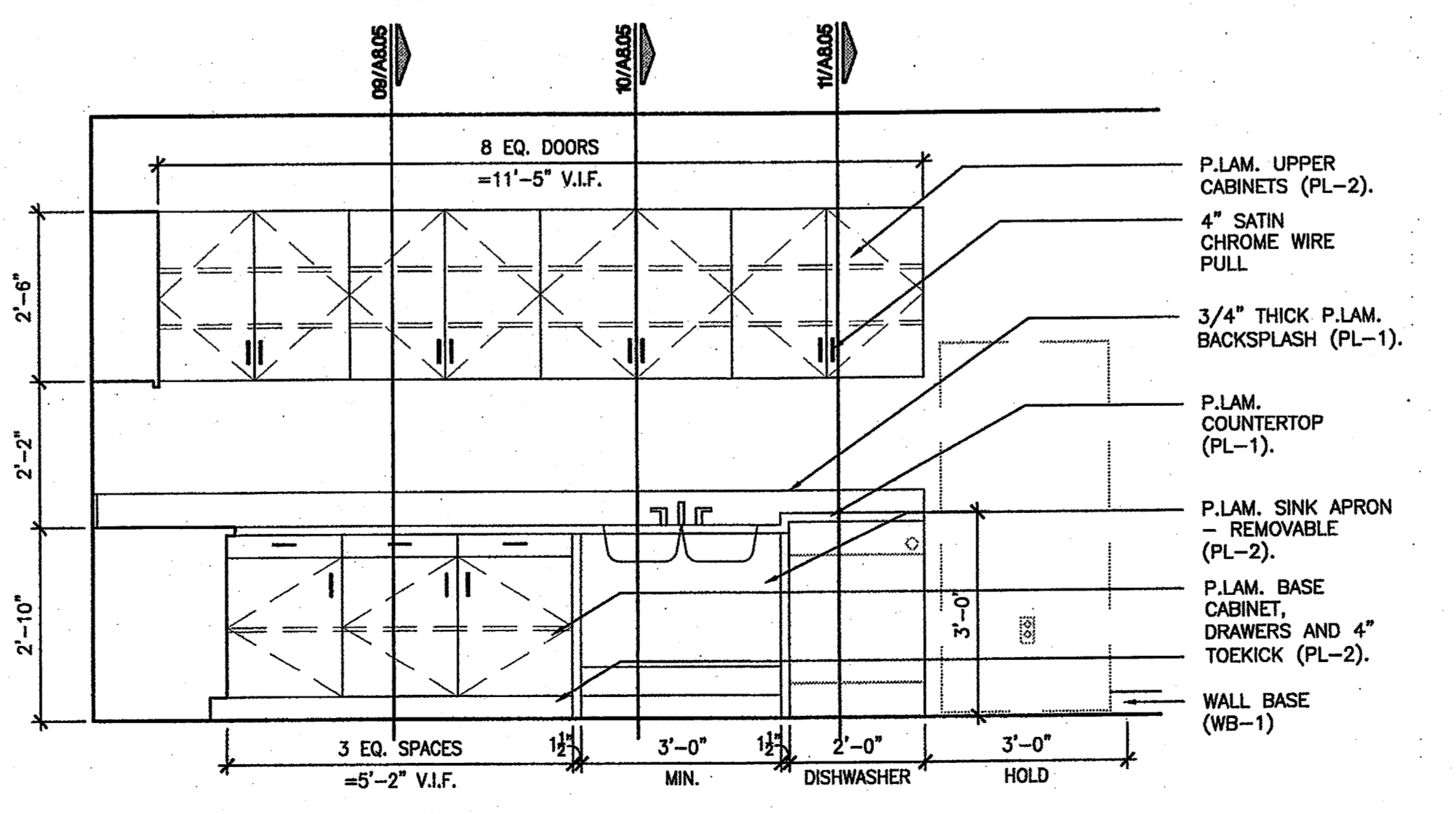
08 RECEPTION ELEV. SCALE: 1/4" = 1'-0"
