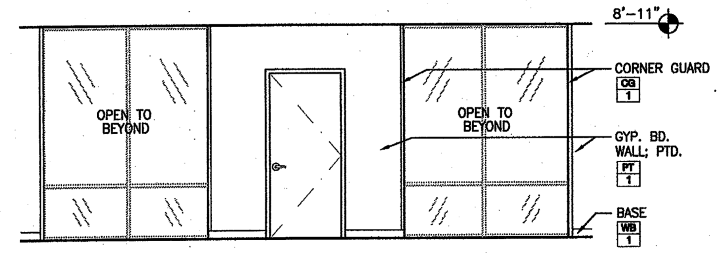
08 RECEPTION ELEV. SCALE: 1/4" = 1'-0"
