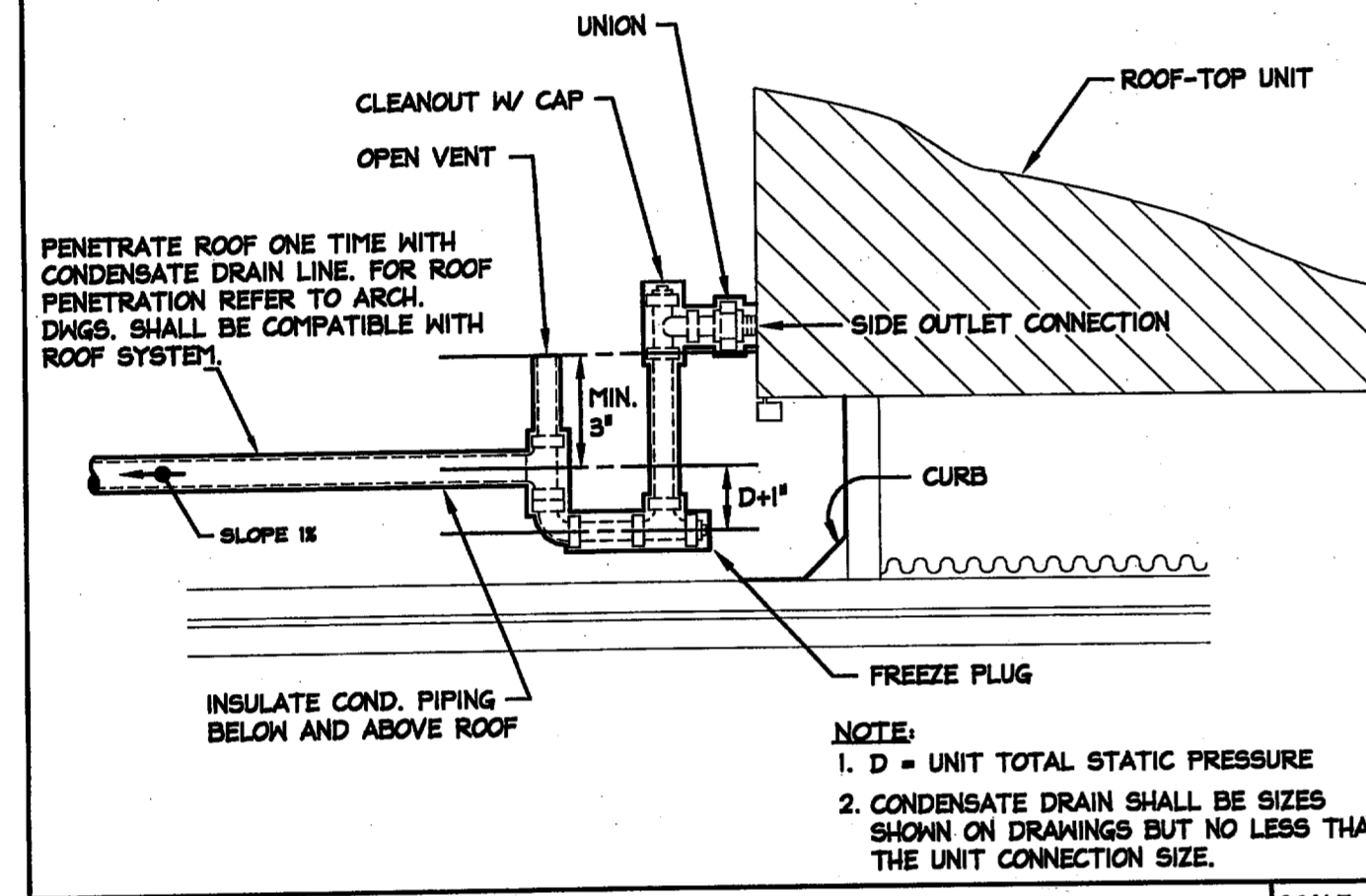
05 ROOFTOP UNIT CONDENSATE PIPING SCALE: NTS
