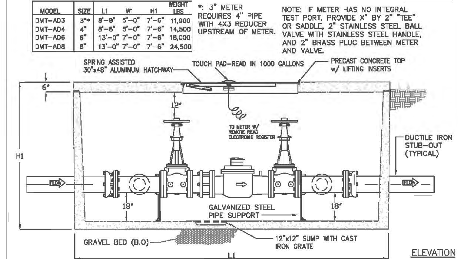
ELEVATION
