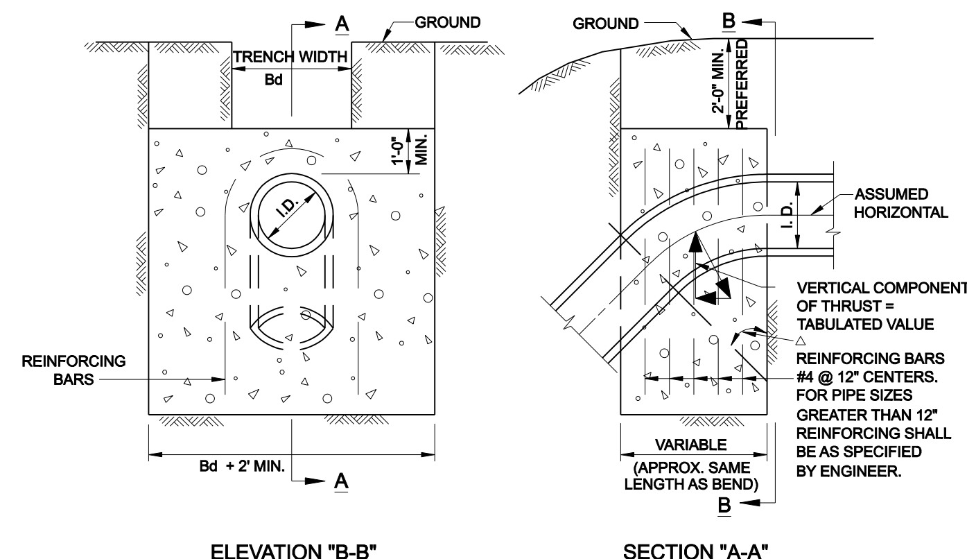
ELEVATION "B-B"
