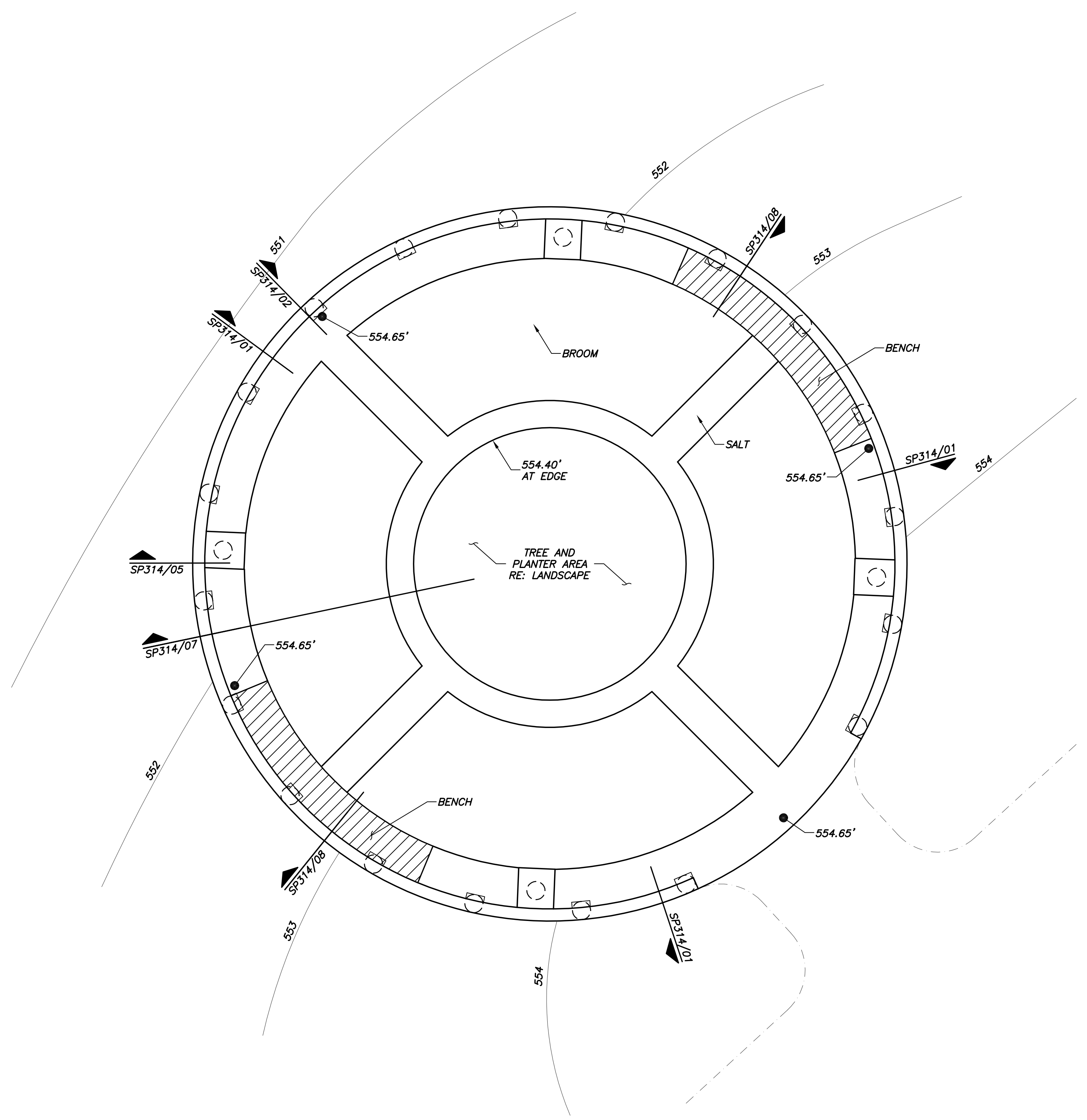
01 BELVEDERE PLAN 1/4"=1'-0"
