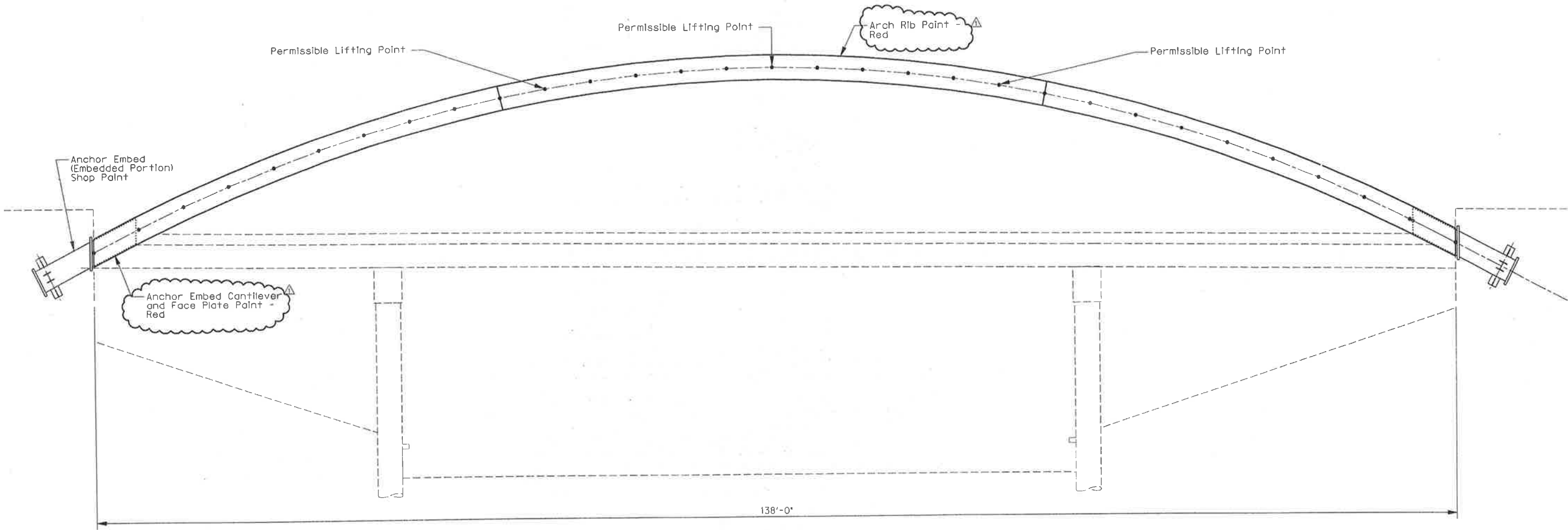
ELEVATION SCALE: 3/16" = 1'-0"
