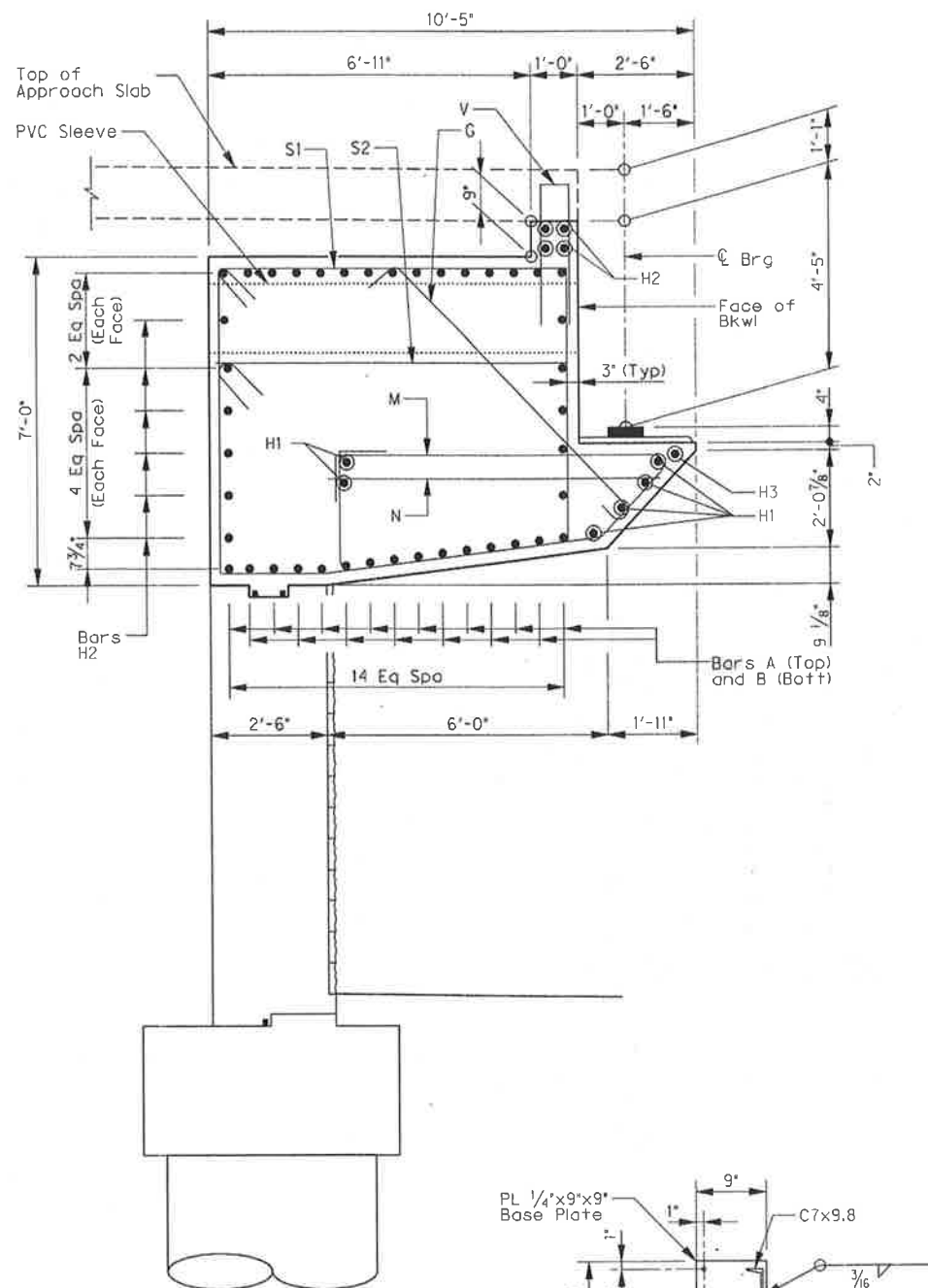
SECTION A-A (CAP) SCALE: 1/2" = 1'-0"
