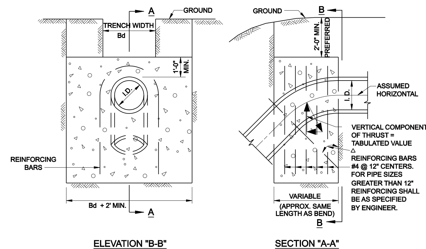
ELEVATION "B-B"
