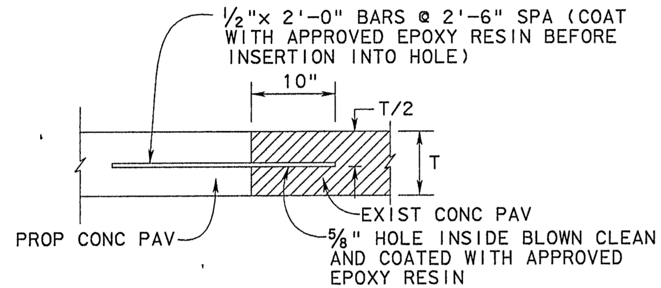
ANCHOR JOINT DETAIL N.T.S.
